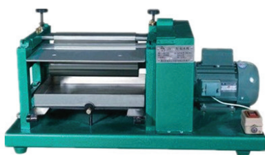
RTGM460
